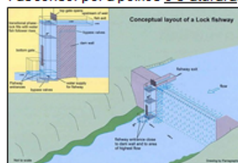
Enclusa per a peixos segons Thomcraft & Harris (2000).
